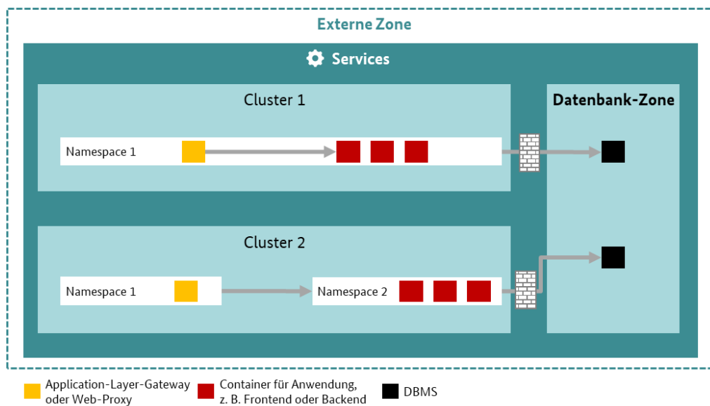
Abbildung 9: Weiche Trennung der Container-Cluster in Externer Zone (illustrative Darstellung)
