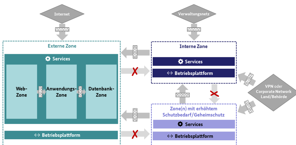
Abbildung 7: Blaupause des einheitlichen Zonenmodells der Cloud-Standorte
